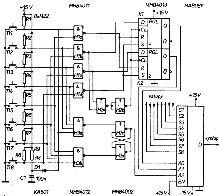
Obr. 4. Schéma zapojení osmikanalového přepínače
